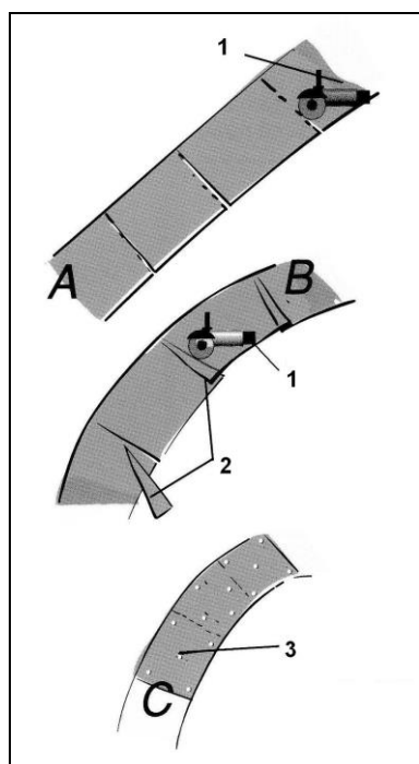
Rys. 4. Układanie siatki na łuku poziomym
