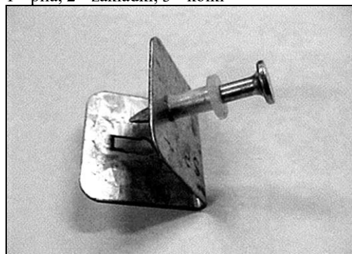
Rys. 5. Klips i kołek do mocowania siatki w podłożu. Klips zakłada się na poprzeczny pręt płaski siatki
